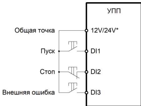
Рисунок 3 – Двухпроводная и трехпроводная схема управления
